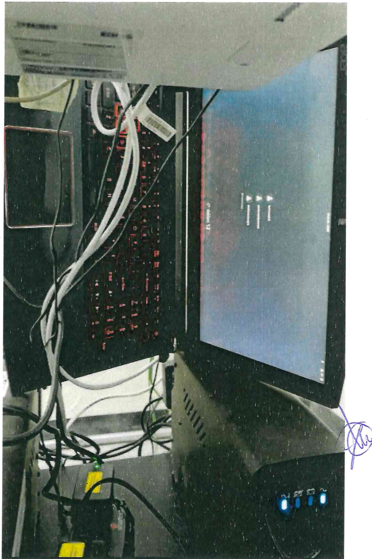
Laptop adaptada para realizar funciones de Servidor Web
